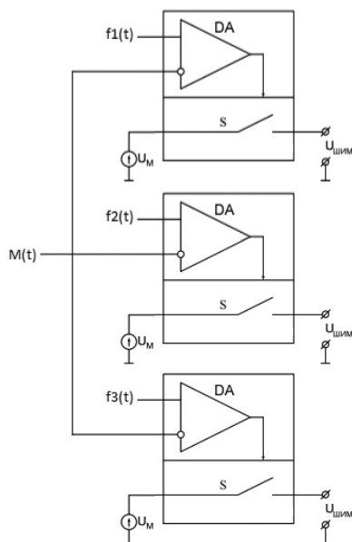
Рисунок 3. Трехканальный ШИМ-контроллер Источник: разработано автором на основе [6]
